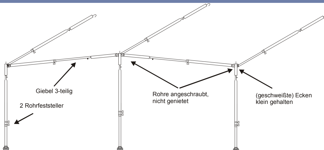
Grundaufbau eines Stahlgerüsts
